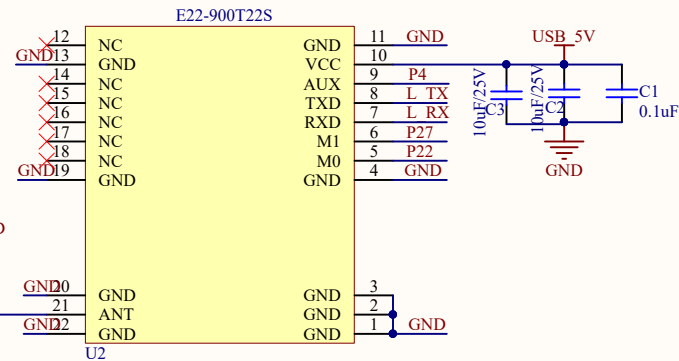
LoRa Module
