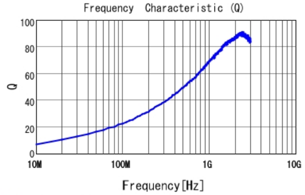
■ LQW15AN15NJ00 Q
