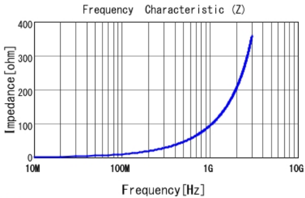
■ LQW15AN15NJ00 |Z|
