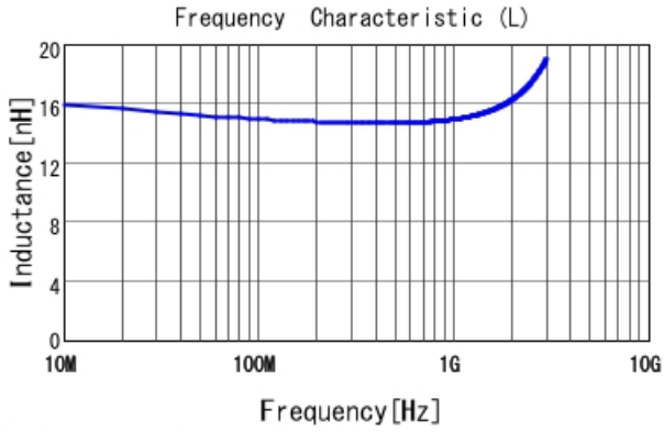
■ LQW15AN15NJ00 L
