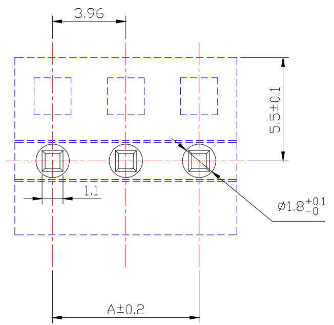
P.C.B LAYOUT
