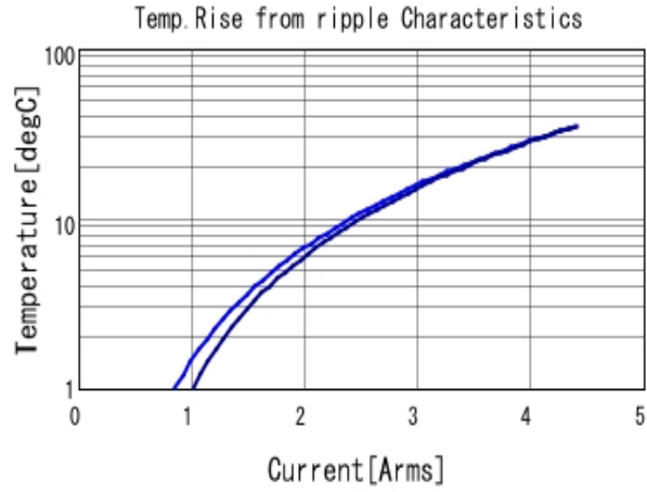
■ GRT188R61E475KE13 Temp. rise ■ 500kHz ■ 1MHz
