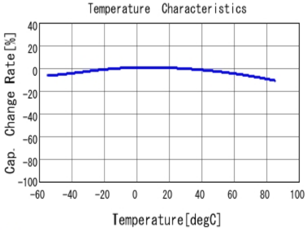
■ GRT188R61E475KE13 C-Temp. capchange, DCO. 0V, ACO. 5V rm
