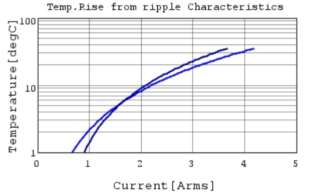
GCM21BR71H105KA03 Temp.rise — 500kHz
