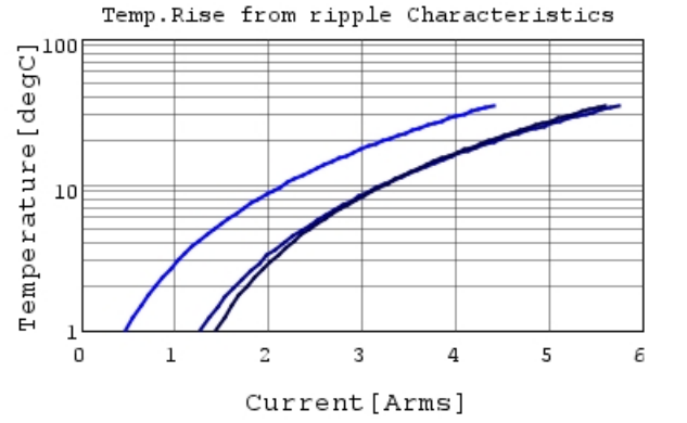
GRM21BR61A226ME51 Temp.rise — 80kHz —
