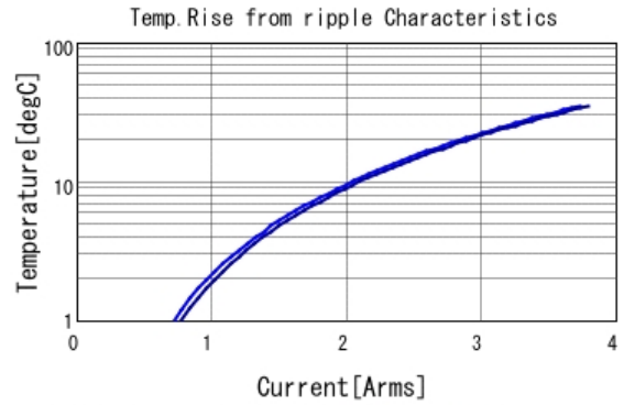
GRT188R61H225KE13 Temp. rise ■ 500kHz ■ 1MHz
