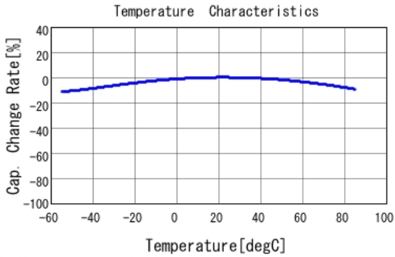
■ GRT188R61H225KE13 C-Temp. capchange, DCO. 0V, ACO. 5Vrm
