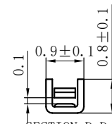
SECTION D-D
